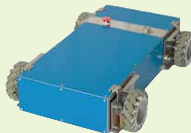
台車にも応用できる全方向移動型「メカナムロボット」
